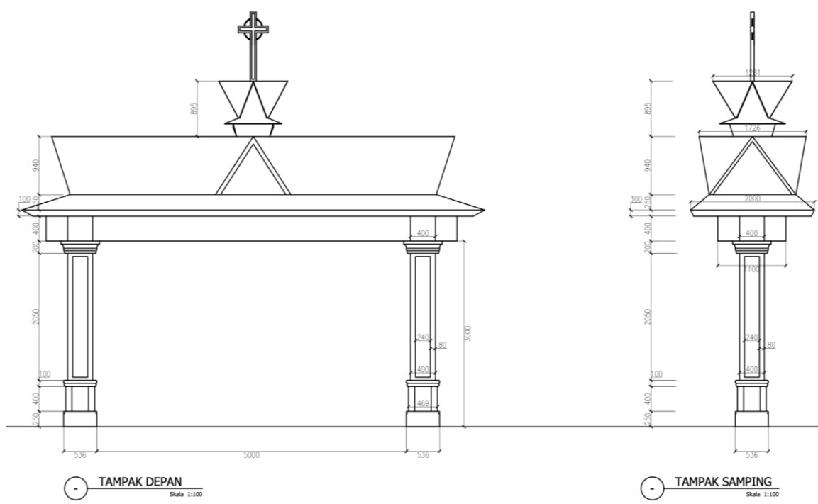
Gambar 6. Tampak Gapura Gereja
