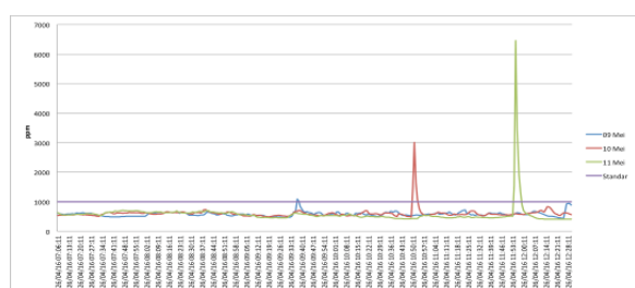
Gambar 2. Grafik Konsentrasi CO 2 , Sudut Inklinasi Jendela 30°
