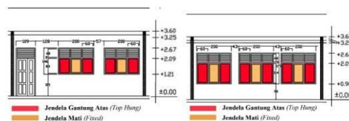
Gambar 2. Tipe Jendela
