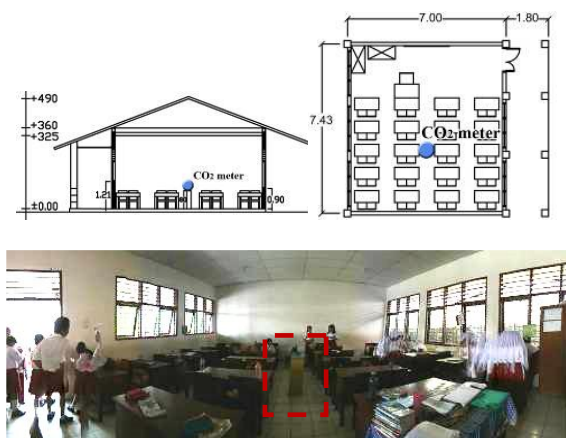
Gambar 3. Perletakan Alat Ukur.
