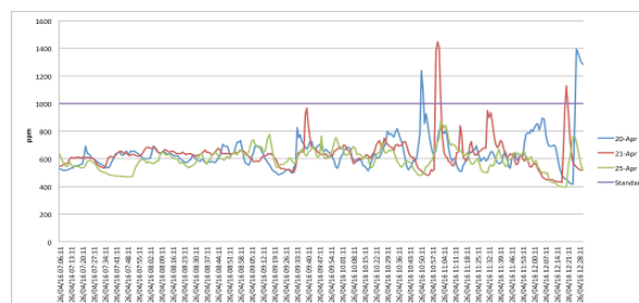
Gambar 4. Grafik Konsentrasi CO 2 , Sudut Inklinasi Jendela 10°
